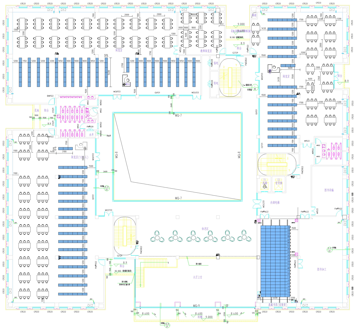
三楼平面布置
